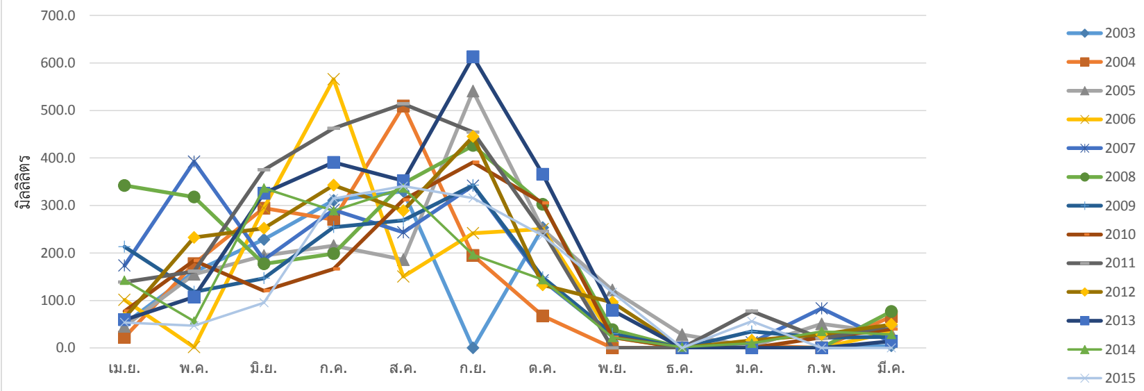
กราฟน้ำฝนรายเดือน สถานี kgt.14
